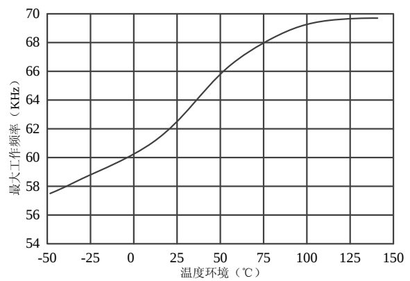
图 3.4 最大工作频率 VS 温度
