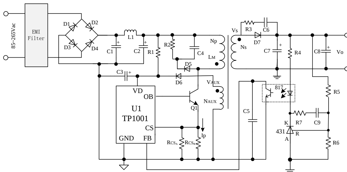
图 8 12V/1A 电源适配器原理图
